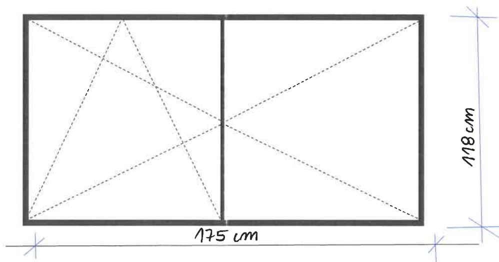
Schemat jednego okna w budynku nr 7 w Świnoujściu
